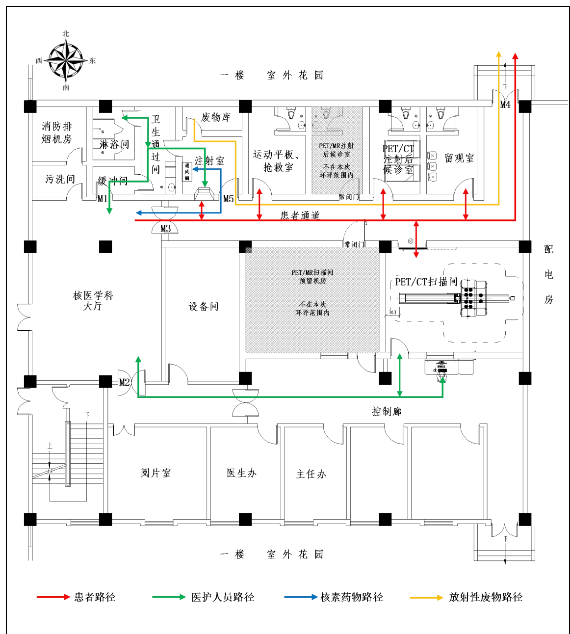
图 9-4 核医学科工作场所布局及病人、医护人员流动路线图
