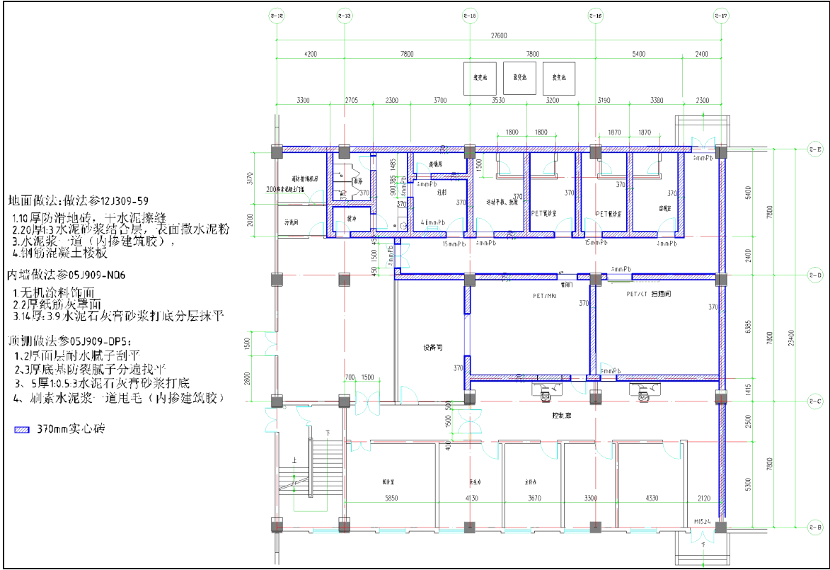
图 10-1 核医学科工作场所屏蔽设计图
