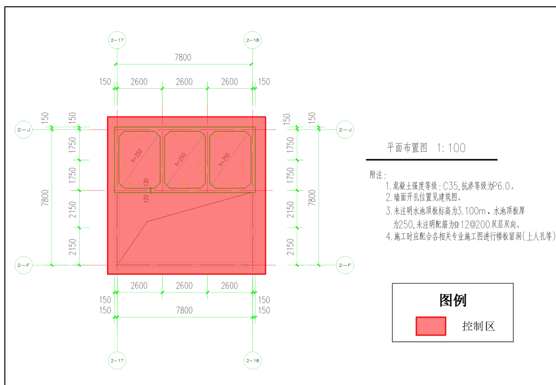
图 10-2 衰变池平面结构示意图
