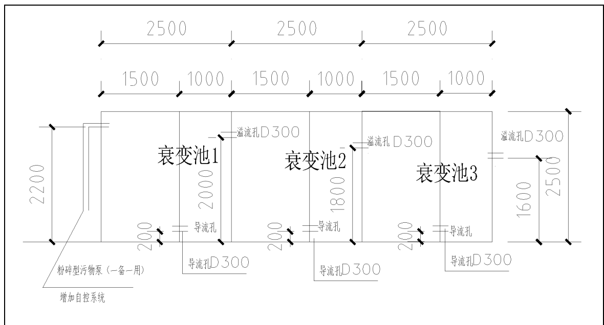
图 10-3 衰变池立面结构示意图
