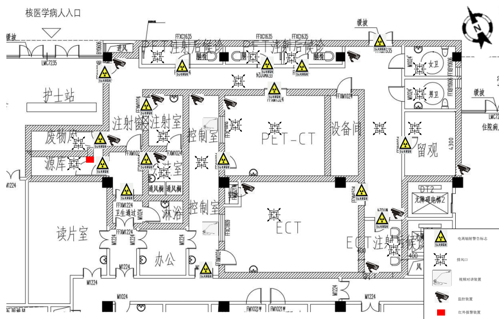
图 10-1 PET/CT 工作辐射防护设施平面布置示意图
