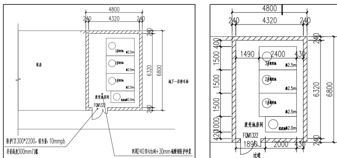
图 10-2 本项目衰变系统结构示意图
