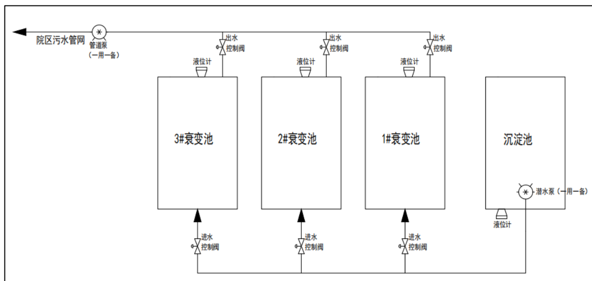
图 10-3 本项目衰变系统工作原理简易示意图
