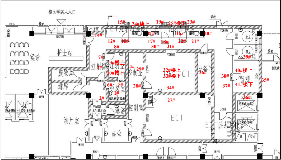
图 11-1 本项目核医学场所剂量率估算点位示意图
